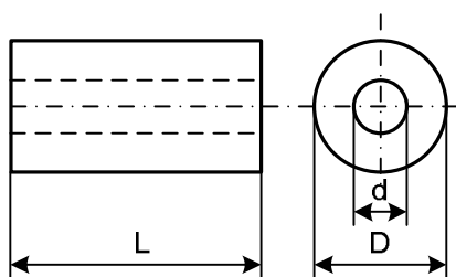
Дисковый керамический коаксиальный резонатор КРД
