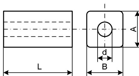
Прямоугольный керамический коаксиальный резонатор КРП
